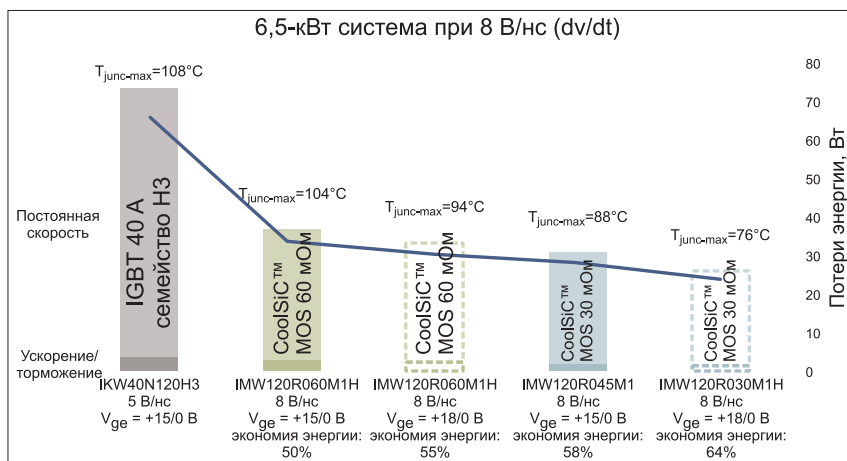
Рис. 4. Сравнение тепловых характеристик и потерь CoolSiC MOSFET с аналогичными показателями высокоскоростных IGBT семейства H3 в случае системы мощностью 6,5 кВт при скорости переключения 8 кВ/мкс в режиме постоянной скорости и ускорения/торможения
