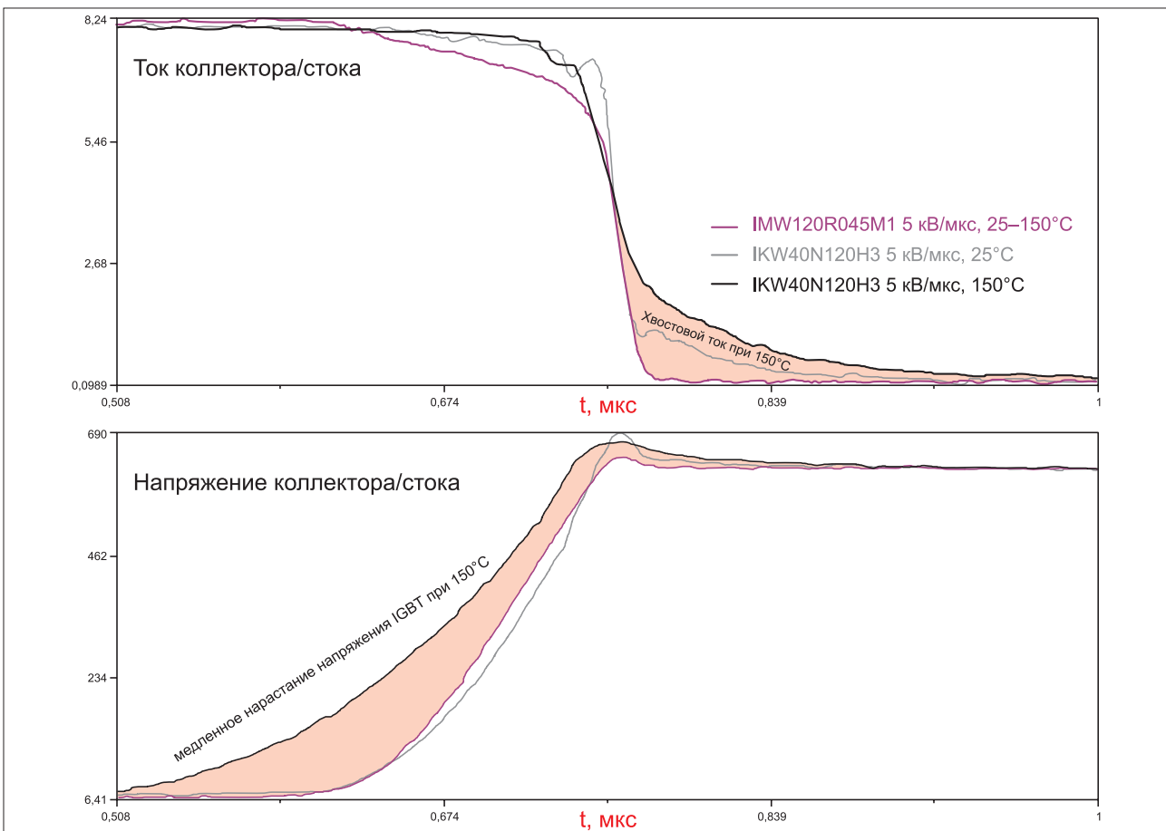
Рис. 2. Сравнение коммутационных характеристик при выключении Si IGBT и CoolSiC MOSFET при 5 кВ/мкс
