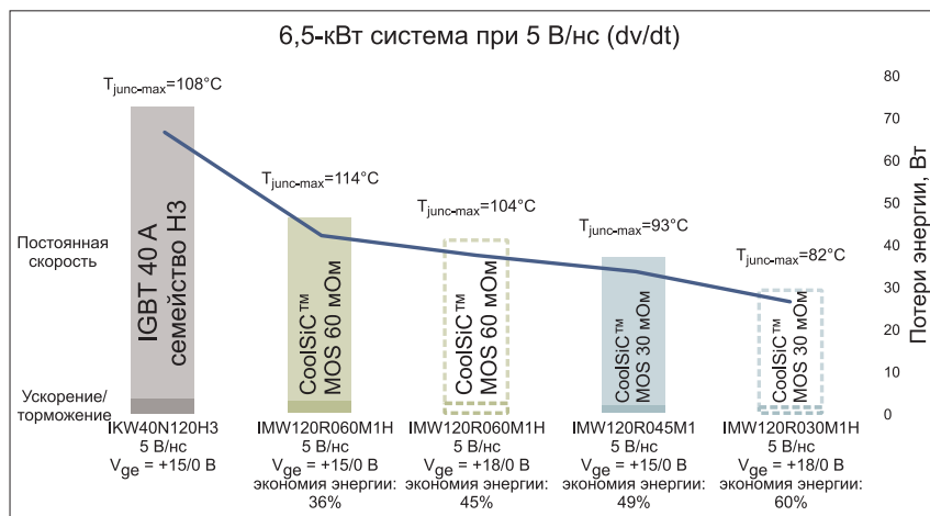
Рис. 3. Сравнение тепловых характеристик и потерь CoolSiC MOSFET с аналогичными показателями высокоскоростных IGBT семейства H3 в случае системы мощностью 6,5 кВт при скорости переключения 5 кВ/мкс в режиме постоянной скорости и ускорения/торможения
