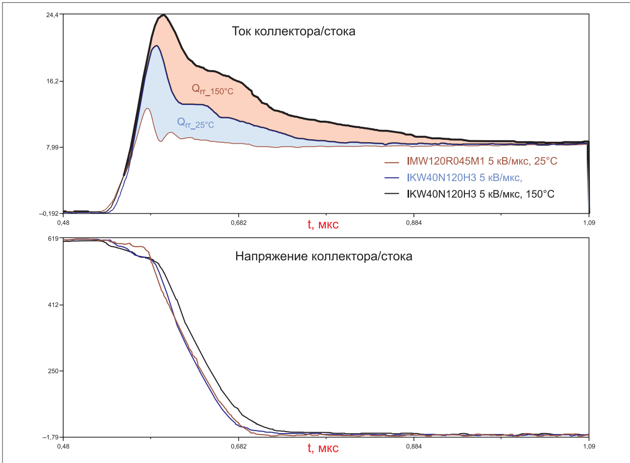
Рис. 1. Сравнение коммутационных характеристик при включении Si IGBT с CoolSiC MOSFET при 5 кВ/мкс
