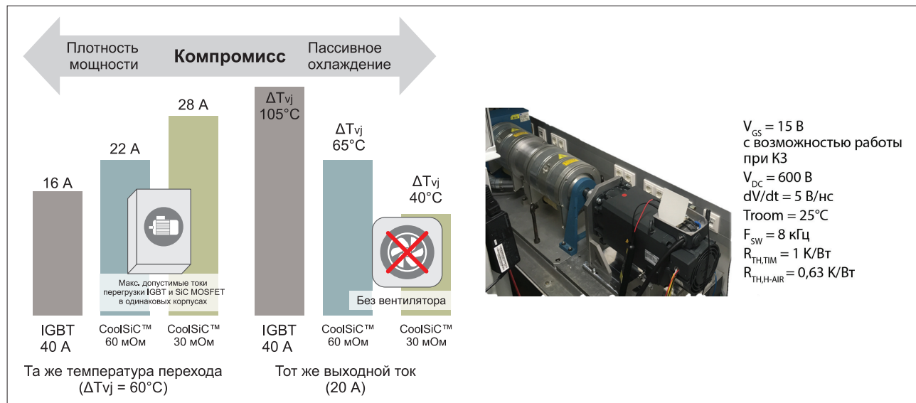
Рис. 5. Пример выбора R_{DS(ON)} с учетом разных требований к сервоприводному решению и вид испытательной установки электродвигателя
