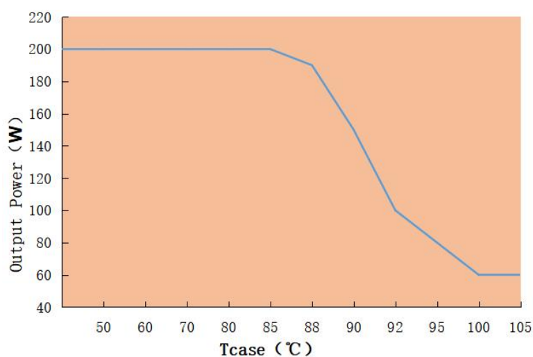
Output power VS Tcase(HVC-200W-56/286)
