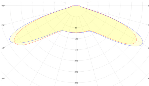
Refond RF-Q50SA40B FWHM = 142°×142°, \eta = 93,1 %
