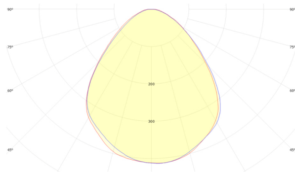
Refond RF-Q50SA40B FWHM = 89°, \eta = 88,7 %
