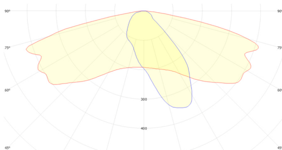
GSLED 5050.V6X.20 FWHM = 157°×47°, \eta = 94,8 %
