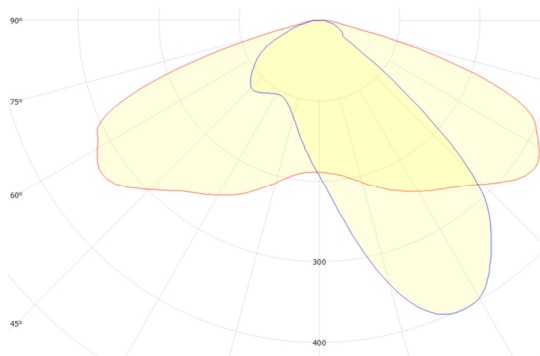
Клевер CLP-5050F5A FWHM = 145°×48°, \eta = 93,1 %
