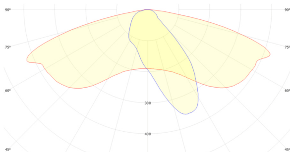
Клевер CLP-5050F5A FWHM = 154°×45°, \eta = 95,2 %
