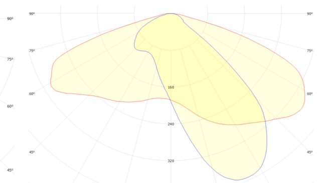
GSLED 5050.V6X.41 FWHM = 144°×48°, \eta = 92,1 %
