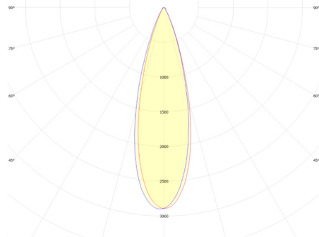
Samsung LH351C FWHM = 29°, \eta = 91,6 %
