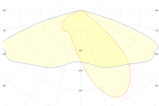
Клевер CLP-5050F5A FWHM = 145°×49°, \eta = 91,1 %
