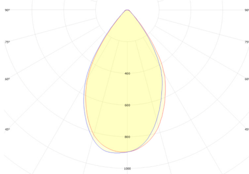
GSLED 5050.V6B.50 FWHM = 62°, \eta = 91,8 %
