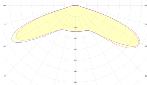
GSLED 5050.V6X.41 FWHM = 142°×143°, \eta = 92,7 %
