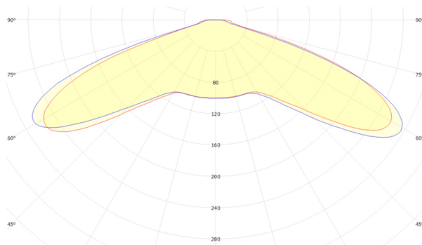
Клевер CLP-5050F5A FWHM = 142°×142°, \eta = 93,6 %
