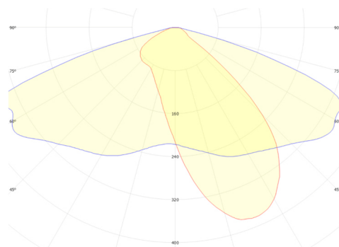
GSLED 5050.V6X.41 FWHM = 146°×49°, \eta = 90,6 %
