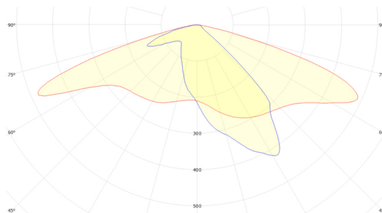
GSLED 5050.V6X.41 FWHM = 147°×47°, \eta = 95,5 %
