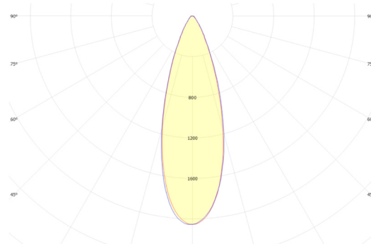
GSLED 5050.V6X.41 FWHM = 33°, \eta = 90,4 %
