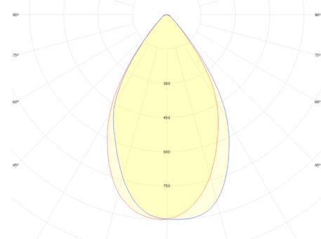
OSRAM DURIS S8 FWHM = 61°, \eta = 92,3 %
