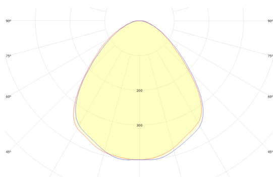
GSLED 5050.V6X.40 FWHM = 92°, \eta = 89,1 %
