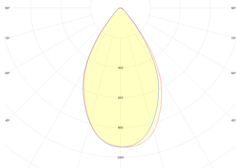
Refond RF-Q50SA40B FWHM = 62°, \eta = 92,4 %
