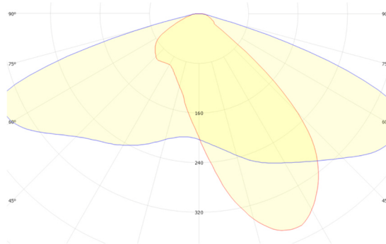
Refond RF-Q50SA40B FWHM = 144°×48°, \eta = 90,2 %
