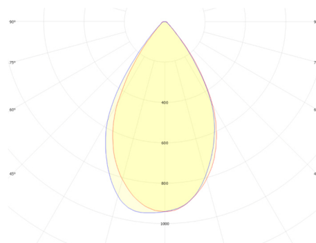
GSLED 5050.V6X.20 FWHM = 60°, \eta = 92,6 %
