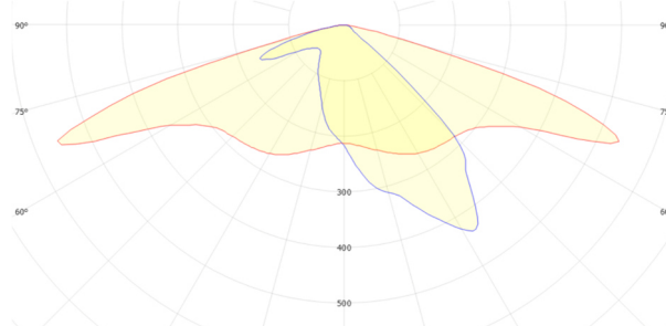
GSLED 5050.V6X.20 FWHM = 147°×47°, \eta = 96,6 %
