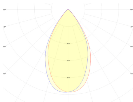
Клевер CLP-5050F5A FWHM = 59°, \eta = 92,7 %
