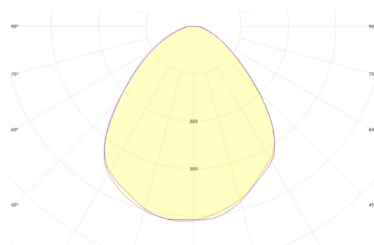
GSLED 5050.V6X.41 FWHM = 90°, \eta = 89,3 %
