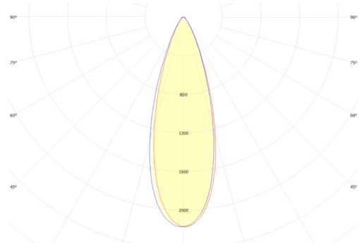
GSLED 5050.V6X.40 FWHM = 33°, \eta = 90,4 %
