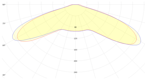
GSLED 5050.V6B.50 FWHM = 144°×144°, \eta = 90,9 %
