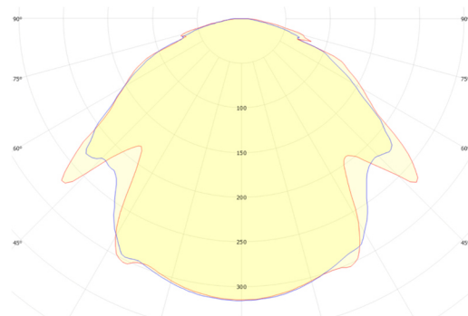
OSRAM DURIS S8 FWHM = 118° × 117°, η = 93,8 %
