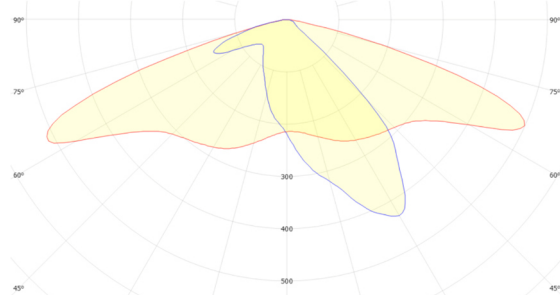
Клевер CLP-5050F5A FWHM = 145°×45°, \eta = 96,4 %
