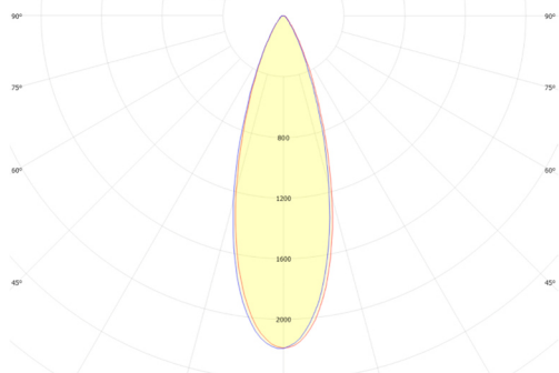
Refond RF-Q50SA40B FWHM = 33°, \eta = 91,6 %
