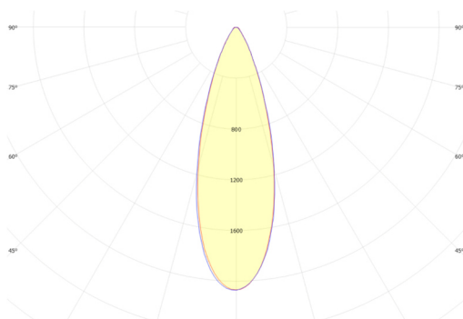
Клевер CLP-5050F5A FWHM = 32°, \eta = 91,2 %
