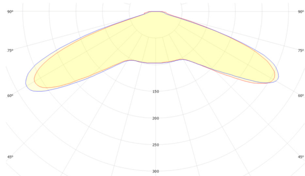
GSLED 5050.V6X.40 FWHM = 142°×142°, \eta = 92,9 %
