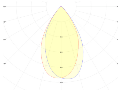
GSLED 5050.V6X.41 FWHM = 60°, \eta = 92,2 %
