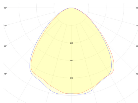
GSLED 5050.V6X.20 FWHM = 94°, \eta = 89,9 %
