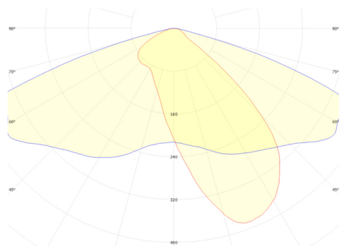
GSLED 5050.V6X.40 FWHM = 145°×49°, \eta = 90,5 %
