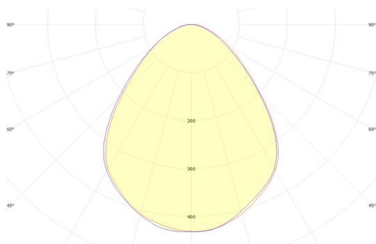
Клевер CLP-5050F5A FWHM = 88°, \eta = 90,1 %
