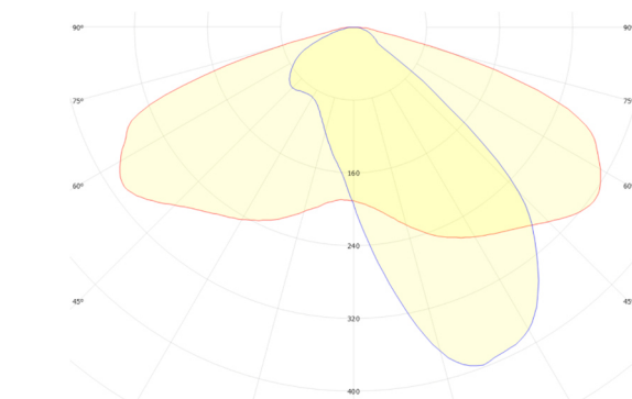
GSLED 5050.V6B.50 FWHM = 145°×48°, \eta = 90,9 %
