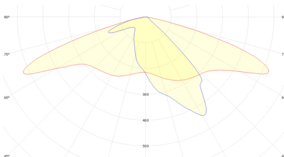
GSLED 5050.V6X.40 FWHM = 146°×45°, \eta = 96,1 %
