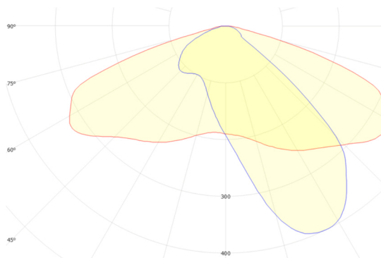
GSLED 5050.V6X.40 FWHM = 145°×48°, \eta = 92,4 %
