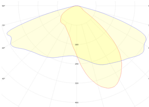
GSLED 5050.V6B.50 FWHM = 146°×50°, \eta = 88,4 %
