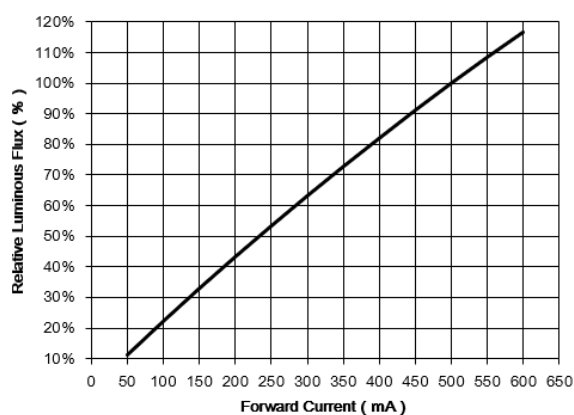
Forward Current Vs. Relative Intensity 正向电流与相对光通量特性曲线
